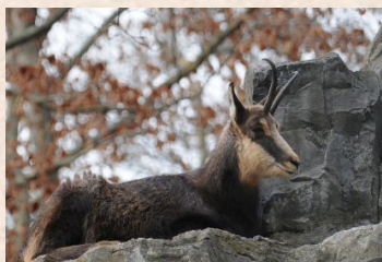
Gems (Europa)
